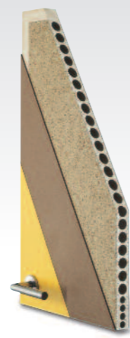
Delikli Okal Levha Azaltılmış delik çapı
